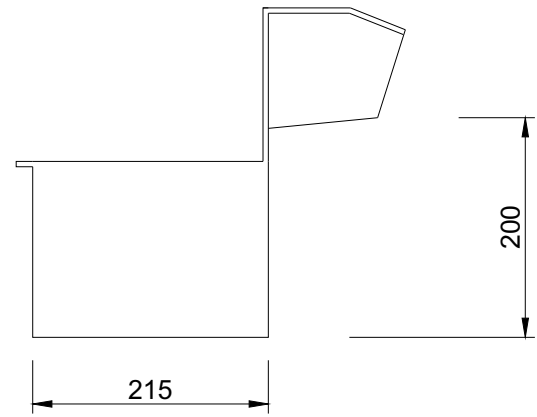
VISTA LATERAL
